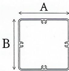
SC6060 SC8080 STAFFA CENTRALE
